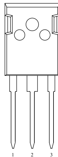
TO247
